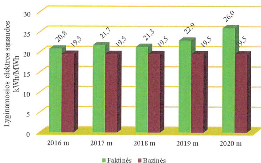
9 pav. UAB „Šakių šilumos tinklai“ faktinių lyginamųjų elektros sąnaudų palyginimas su bazinėmis kWh/MWh.
