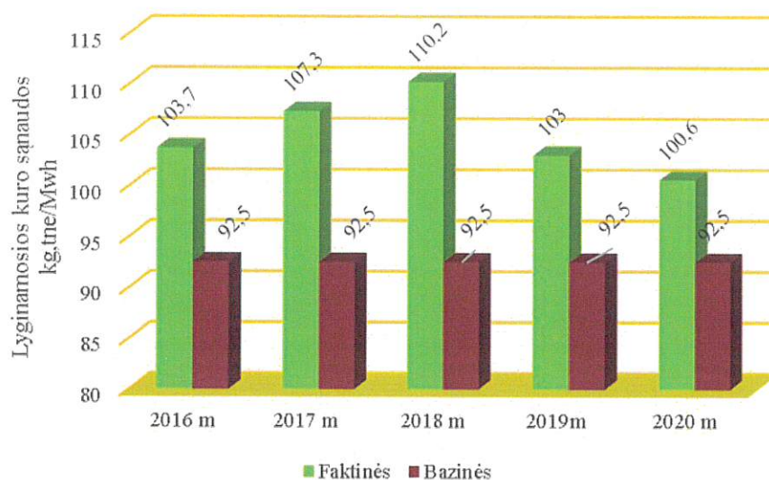
8 pav. UAB „Šakių šilumos tinklai“ faktinių lyginamųjų kuro sąnaudų palyginimas su bazinėmis kg tne/MWh.
