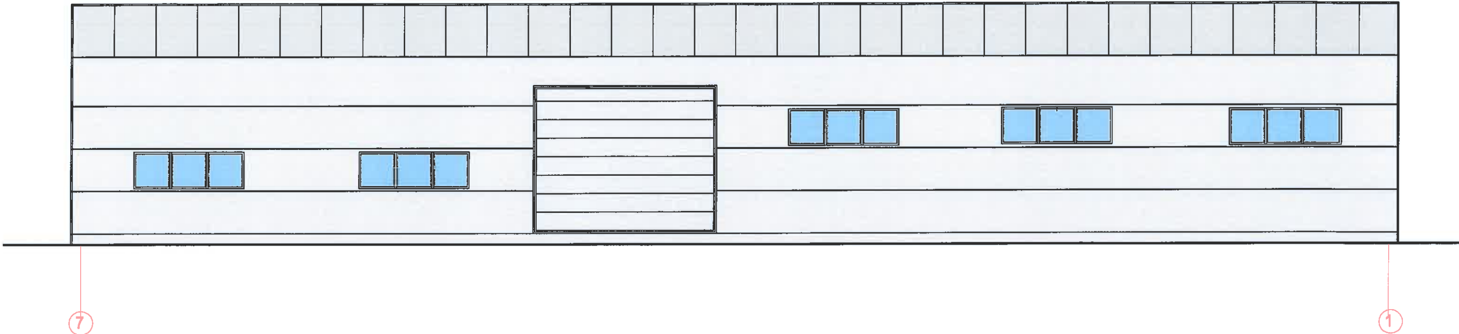
ŠIAURĖS VAKARŲ FASADAS M 1:100
