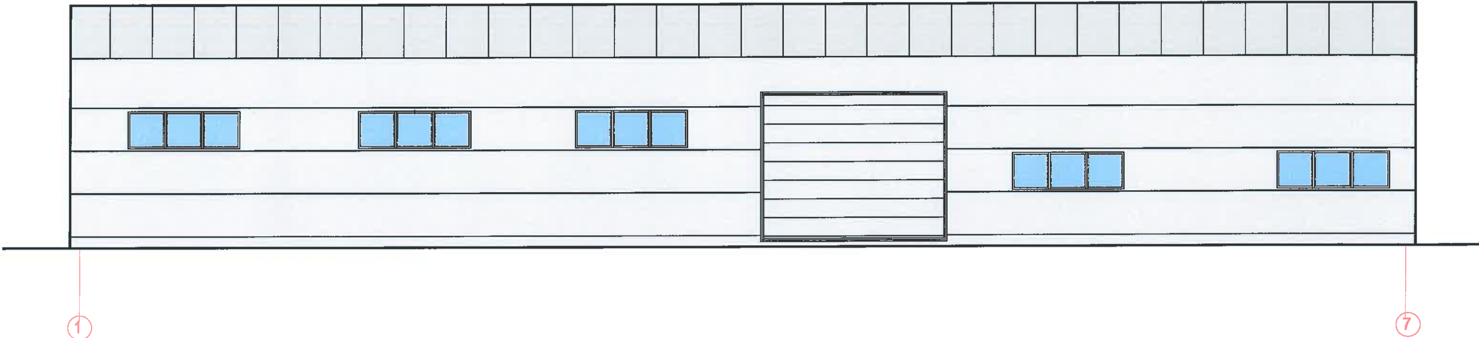
PIETRYČIŲ FASADAS M 1:100
