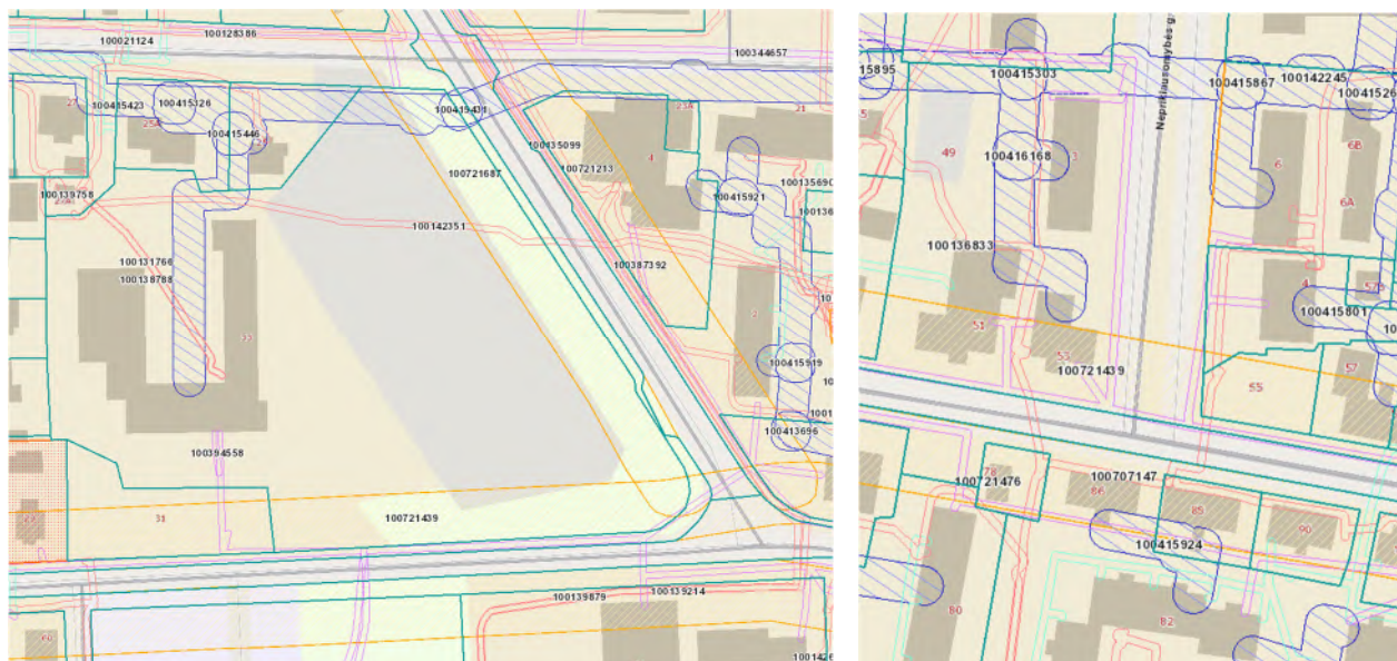
7 pav. Inžineriniai tinklai, sklype Nr. 04 ir Nepriklausomybės g. Ištrauka iš www.regia.lt
