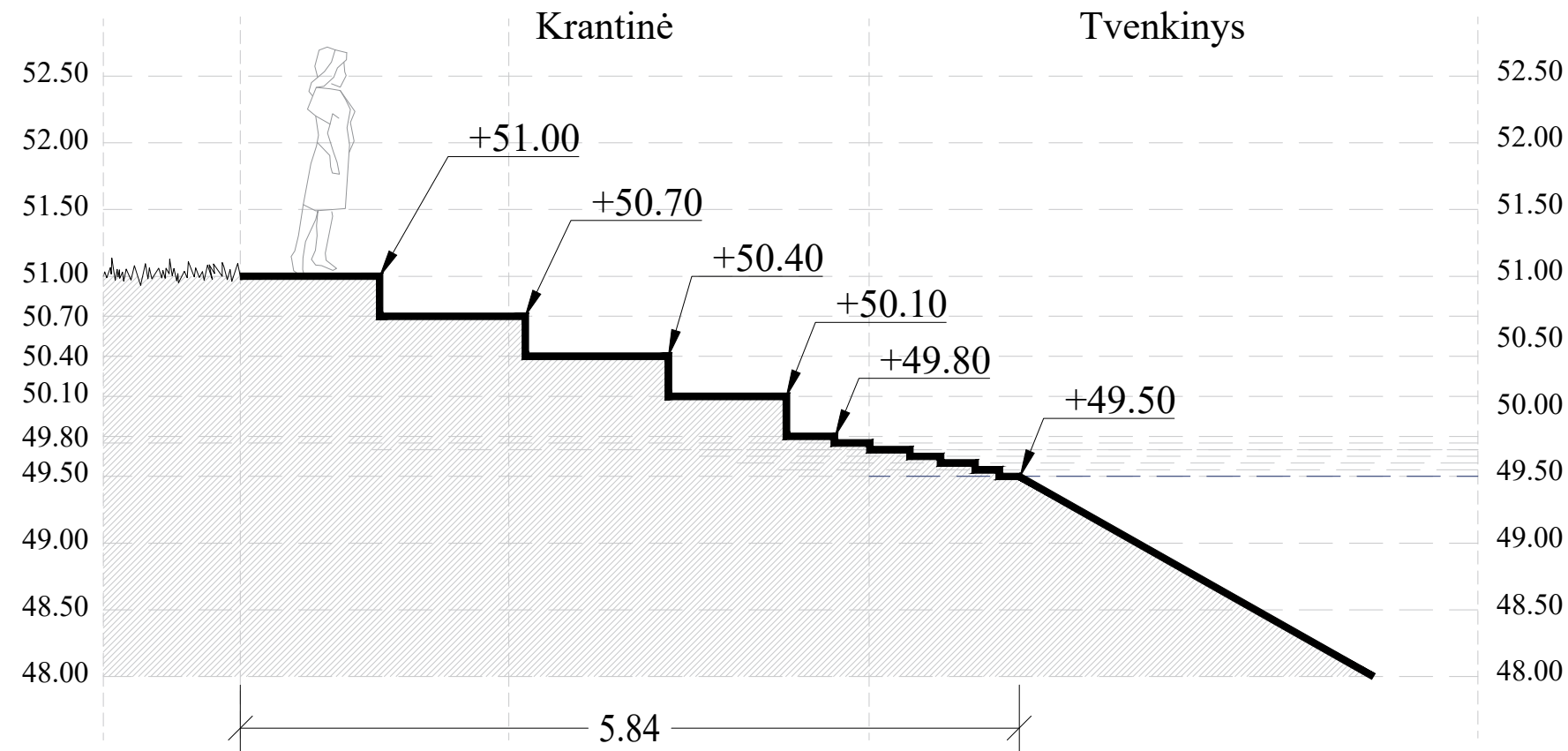
PJŪVIS B-B Principinė krantinės įrengimo schema
