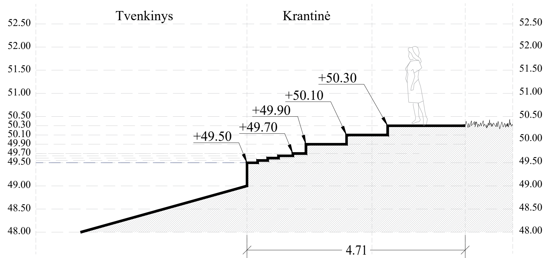
PJŪVIS A-A Principinė krantinės įrengimo schema
