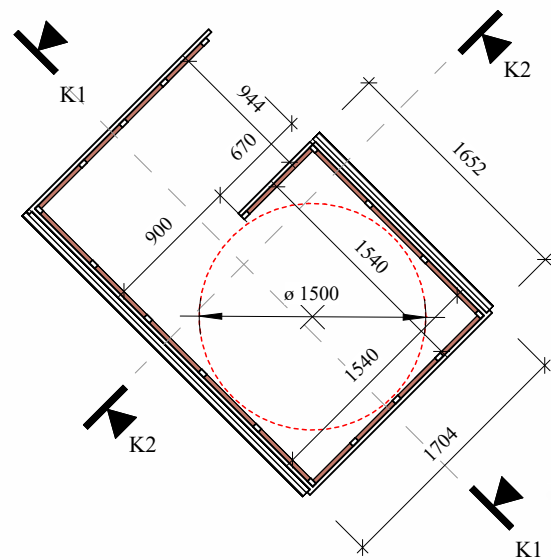
aukšto planas M 1 : 50
