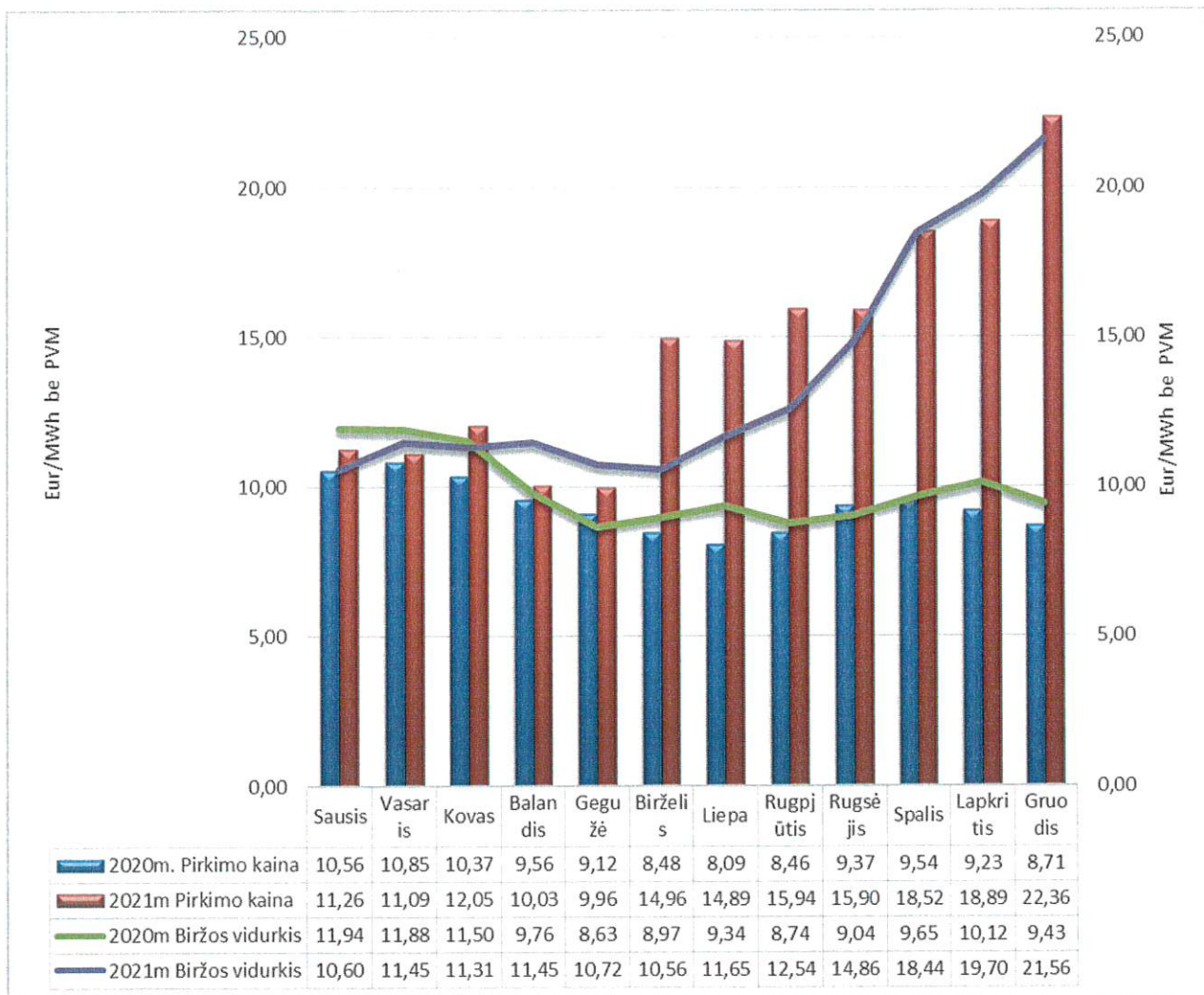
11 pav. UAB „Šakių šilumos tinklai“ 2020 – 2021 m. pirktų kuro (medienos skiedros) kainų dinamika.
