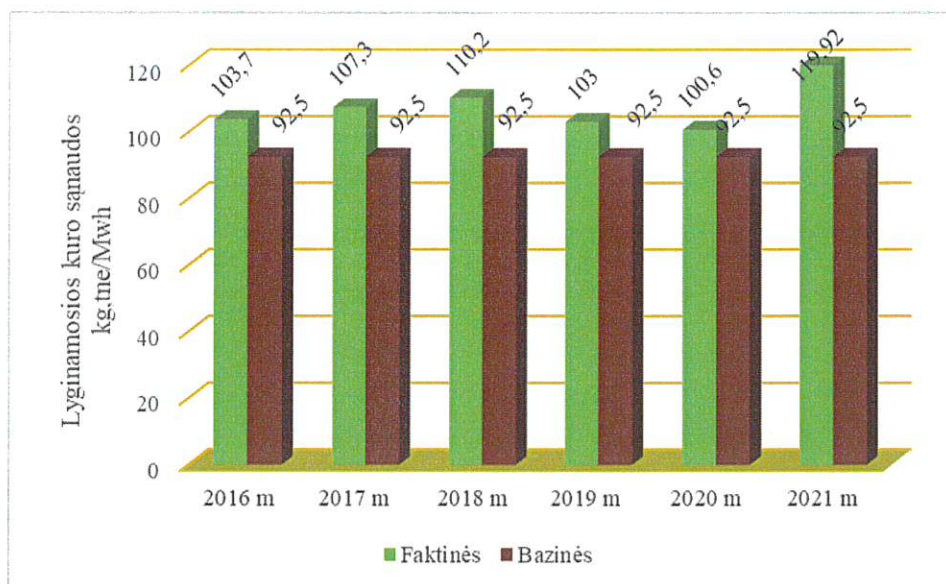
8 pav. UAB „Šakių šilumos tinklai“ faktinių lyginamųjų kuro sąnaudų palyginimas su bazinėmis kg tne/MWh.
