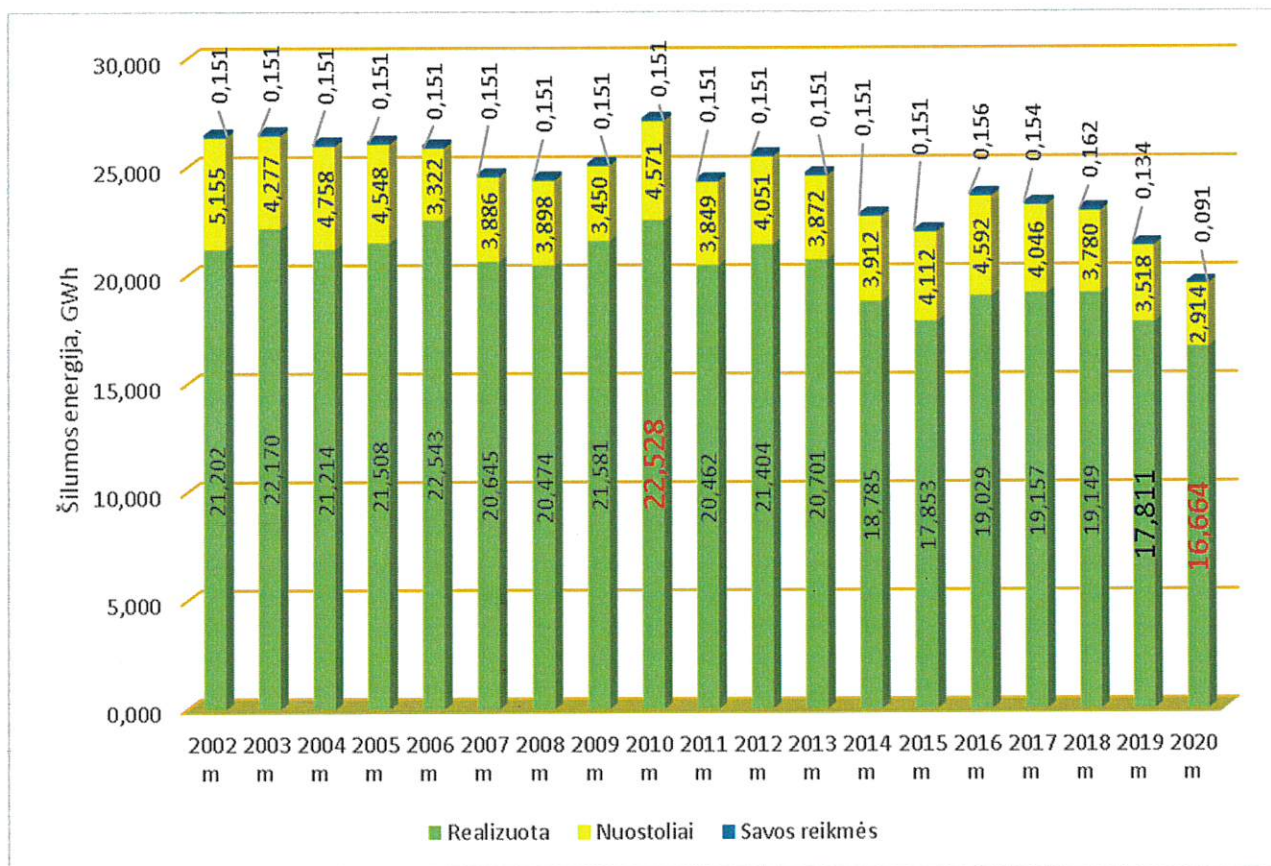
10 pav. UAB „Šakių šilumos tinklai“ 2002 – 2021 m šilumos gamyba.
